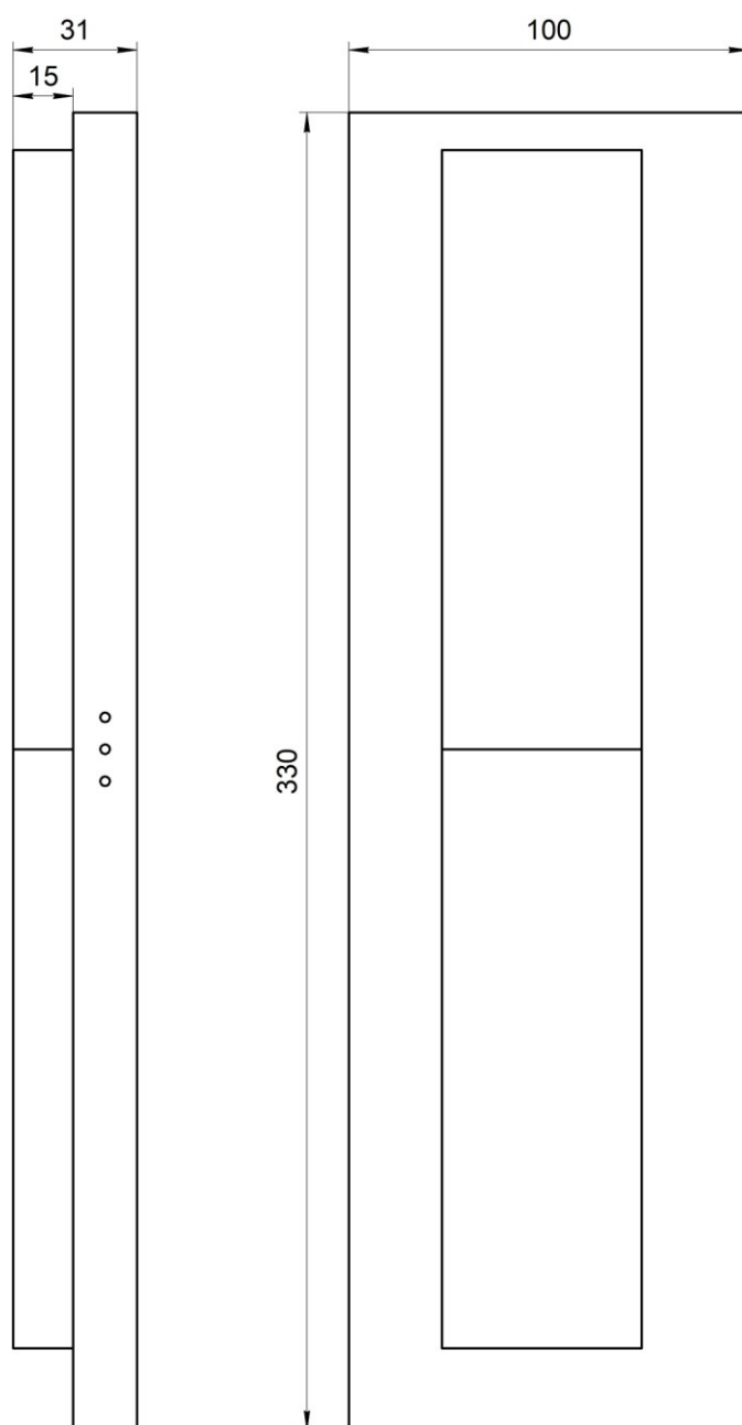
Рис.1 Внешний вид «Указатель лифтовой» НШЕК.468232.205
